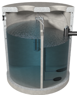
friwa®-klaro Kleinkläranlage
